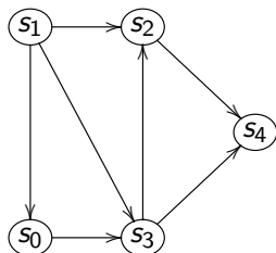
Graphe orienté
