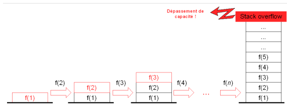
FIGURE – La pile d'exécution de la fonction somme (renommée en f pour raison de concision). (image Developpez.com)
